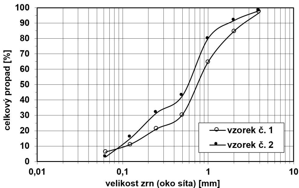
Obr. 8 Příklad grafického vyjádření distribuce velikosti zrn kameniva na základě hodnot celkových propadů jednotlivými sítí při síťovém rozboru, provedeném na dvou vzorcích kameniva z vápenných omítek (kumulativní zrnitostní křivky).
